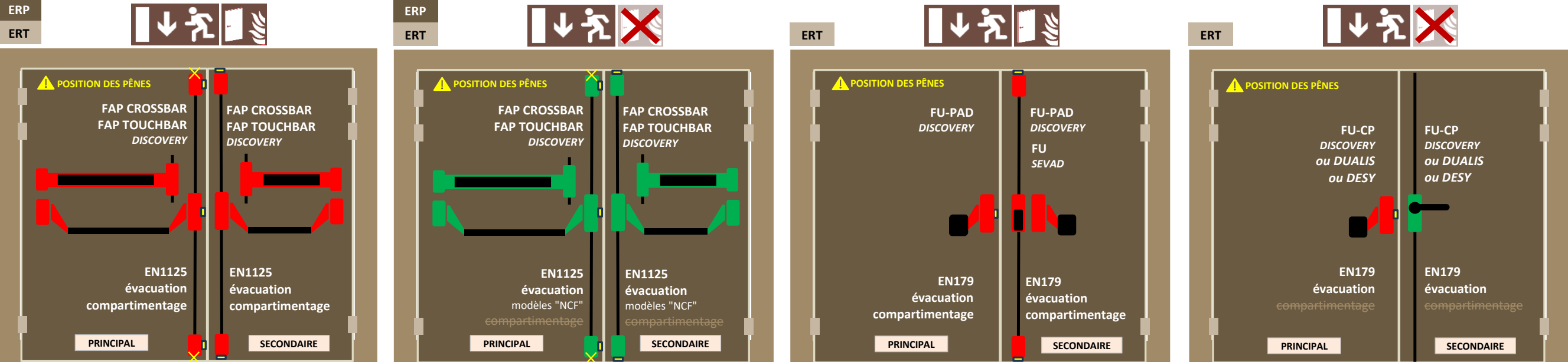
Bloc-Porte 2 vantaux, coupe-feu et issue de secours pour les 2 vantaux ( en ERP et/ou en ERT) Bloc-Porte 2 vantaux, non coupe-feu et issue de secours pour les 2 vantaux ( en ERP et/ou en ERT) Bloc-Porte 2 vantaux, coupe-feu et issue de secours pour les 2 vantaux ( en ERT uniquement ) Bloc-Porte 2 vantaux, non coupe-feu et issue de secours pour les 2 vantaux ( en ERT uniquement )
