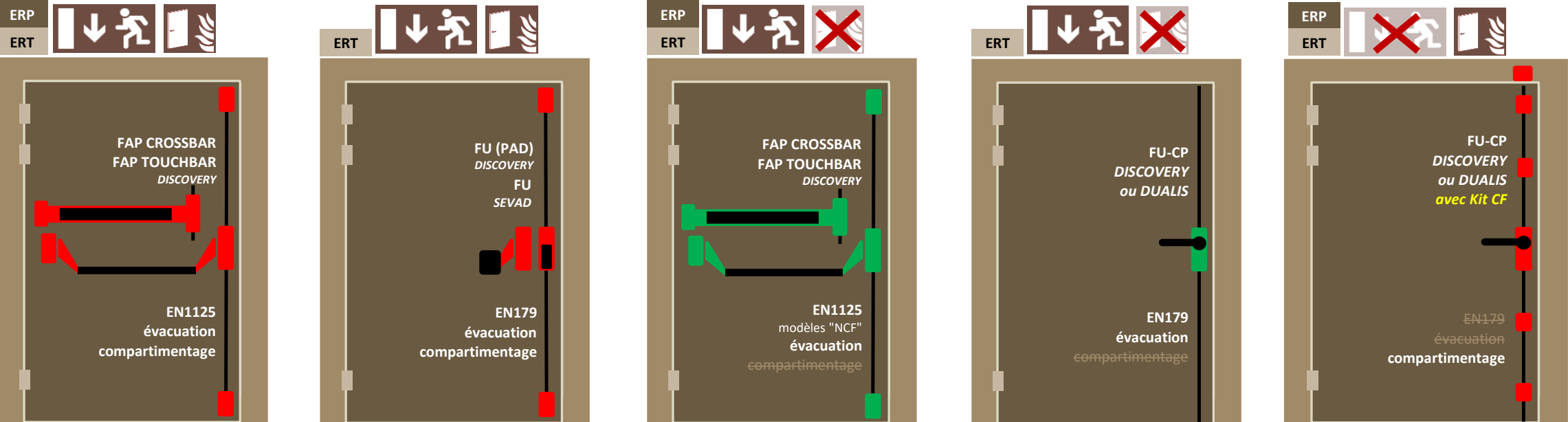
Bloc-Porte 1 vantail, issue de secours et coupe-feu ( en ERP et/ou en ERT) Bloc-Porte 1 vantail, issue de secours et coupe-feu ( en ERT uniquement) Bloc-Porte 1 vantail, issue de secours et non coupe-feu (en ERP et/ou en ERT) Bloc-Porte 1 vantail, issue de secours et non coupe-feu (en ERT uniquement) Bloc-Porte 1 vantail coupe-feu et non située sur issue de secours (en ERP et/ou en ERT)
