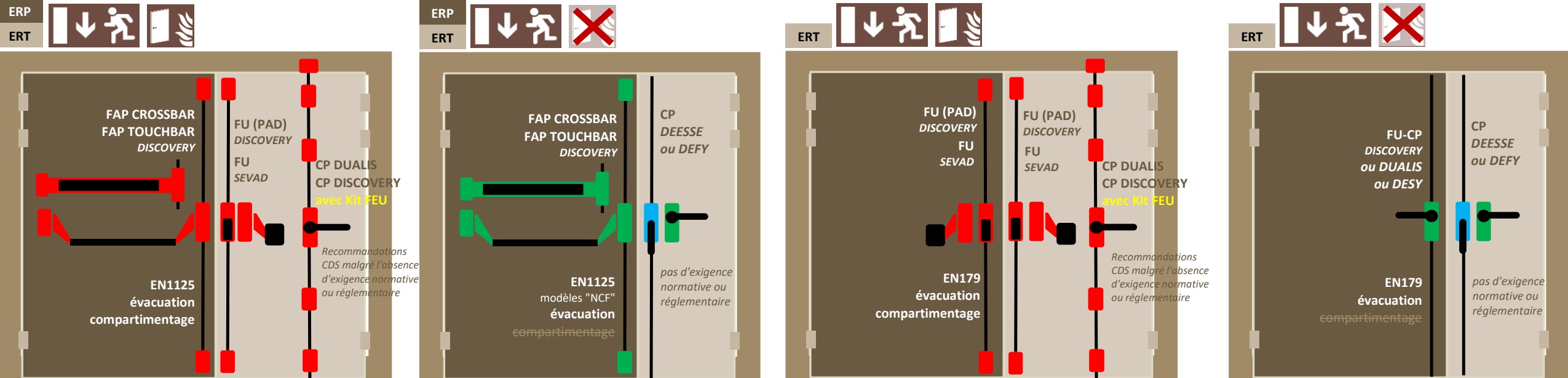
Bloc-Porte 2 vantaux, coupe-feu pour les 2 vantaux et issue de secours pour le vantail principal uniquement ( en ERP et/ou en ERT) Bloc-Porte 2 vantaux, non coupe-feu et issue de secours pour le vantail principal uniquement ( en ERP et/ou en ERT) Bloc-Porte 2 vantaux, coupe-feu pour les 2 vantaux et issue de secours pour le vantail principal uniquement ( en ERT uniquement) Bloc-Porte 2 vantaux, non coupe-feu et issue de secours pour le vantail principal uniquement (en ERT uniquement)
